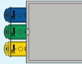
MINI TABS FINGOOD: APF-F858-3 MINIMUM WALL CLEARANCE: 12.5"
