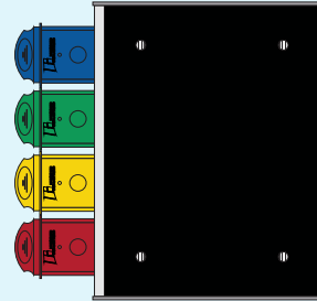
MINI TABS FINGOOD: HIDPF-F8511-4 MINIMUM WALL CLEARANCE: 13"
